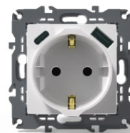
S20.129.10 - Base corriente 16A + 2 USB Tipo A y C 6 UDS 60 UDS PROTECCIÓN INFANTIL
